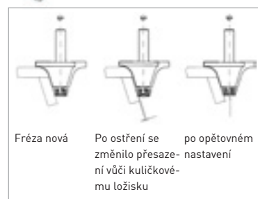
Axiálně posuvné kuličkové ložisko u tvarové frézy pro hrany umyvadel
